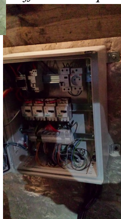
Coffret électrique
